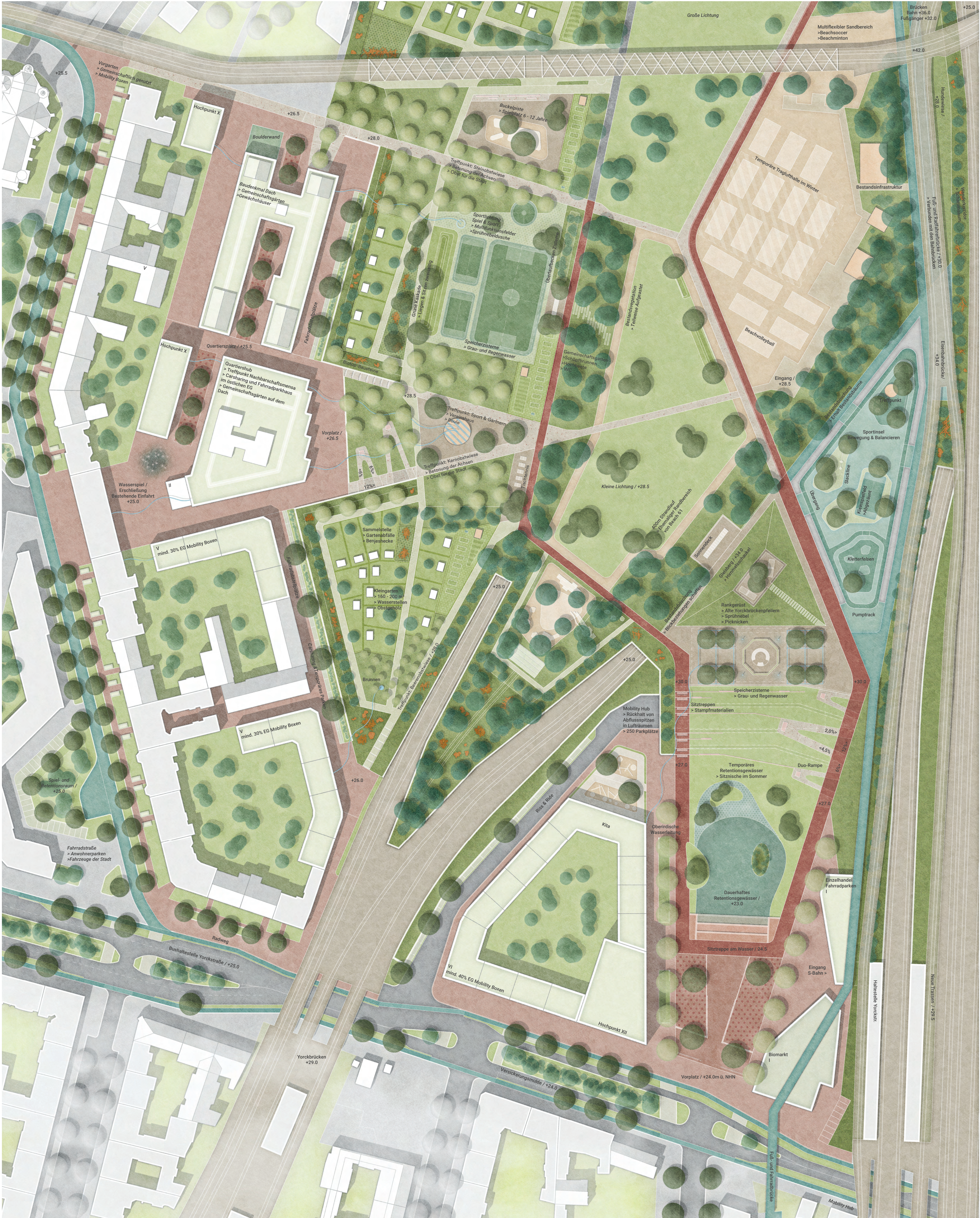
LAGEPLAN M 1:500
