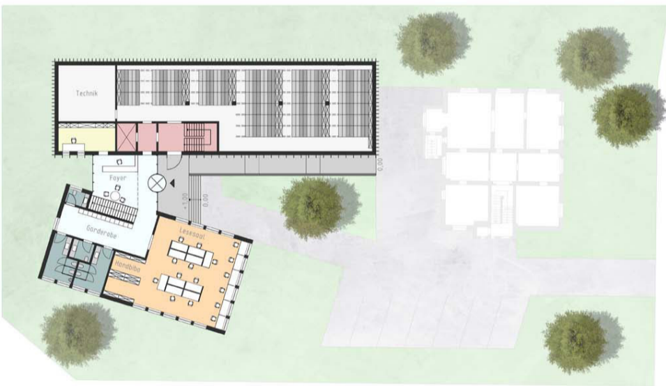
Grundstück mit Grundriss EG M 1:200
